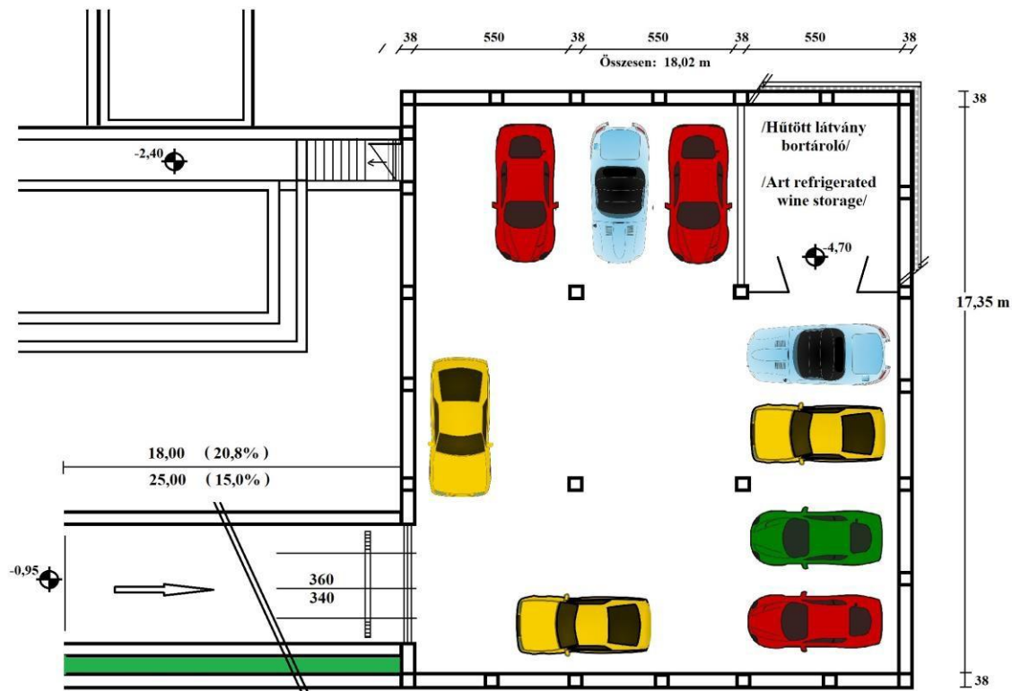
CSALÁDIHÁZ TERV / GARÁZS ALAPRAJZA / 1165 Budapest, Koronafürdő utca 15.
